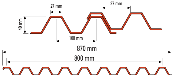
PERFIL ALUBEL 44
