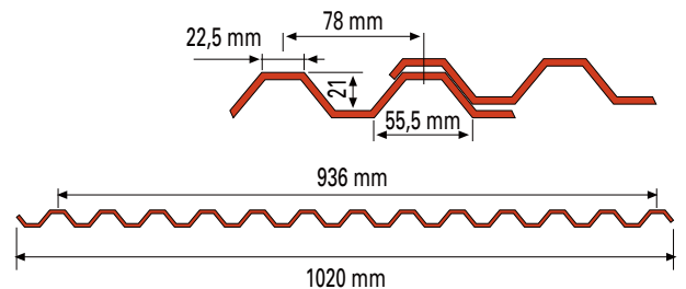
PERFIL ALUBEL 21
