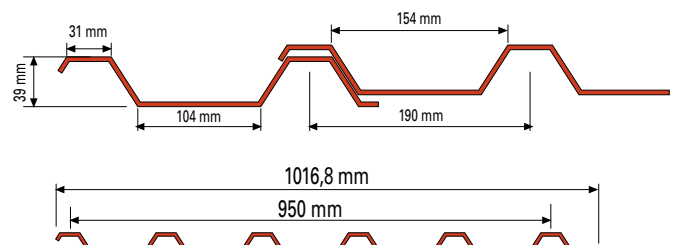
PERFIL ALUBEL 40
