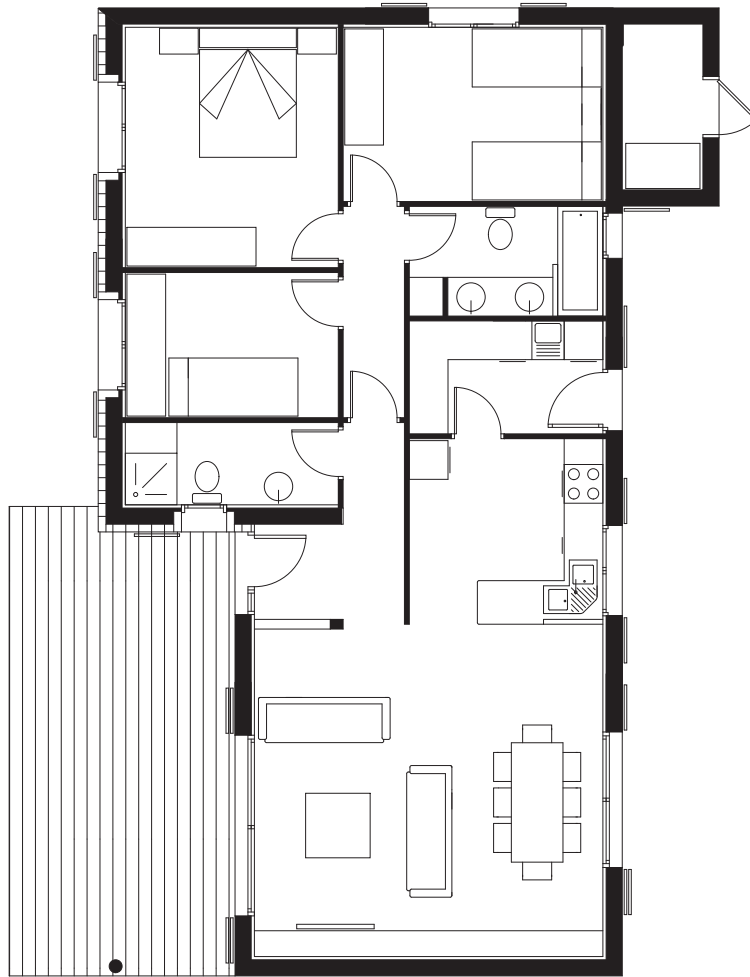
PLANTA BAJA Sup. Construida = 119.11m 2 Sup. Útil = 93.12m 2
