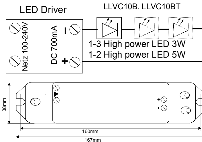
Anschaltbild Circuit diagram Diagrama de circuito
