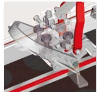
Desplazamiento del cabezal mediante 9 rodamientos
