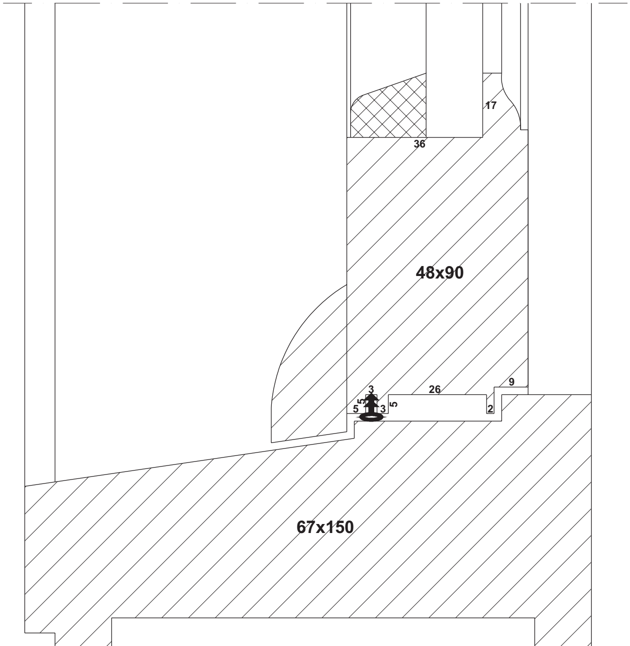
Dibujo E1/1
