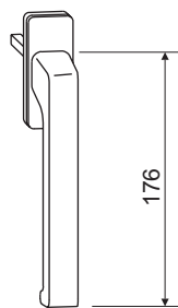
DIRIGENT GRANDE Blanca: 6-31382-40-0-7 Negra: 6-31382-40-0-6 Plata: 6-31382-40-0-11
