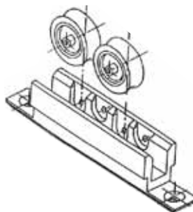
Tándem PVC ventana (2 posiciones Ruedas) VK-43+
