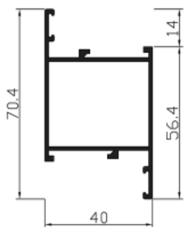
Ref. 10439 Marco puerta con tapajuntas / hoja puerta
