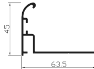
Ref. 65024 Angulo para registro.
