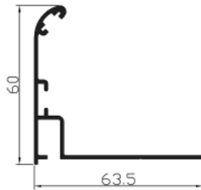
Ref. 65023 Angulo para registro
