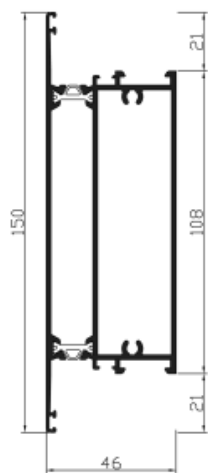
Ref. 22762 Franja / zócalo
