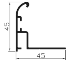
Ref. 65025 Angulo para registro
