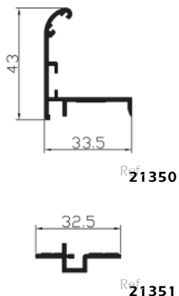
Ref. 21350-21351 21350 -> Angulo para registro. 21351 -> Base para registro.
