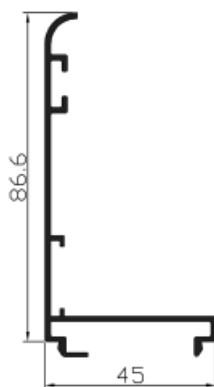
Ref. 24563 Angulo registro 86,6 mm
