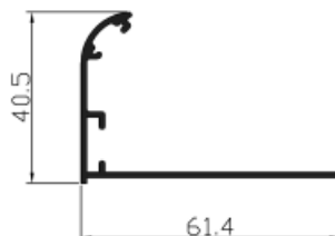
Ref. 65020 Angulo curvo.
