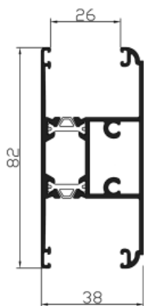
Ref. 22761 Travesaño vidrio directo
