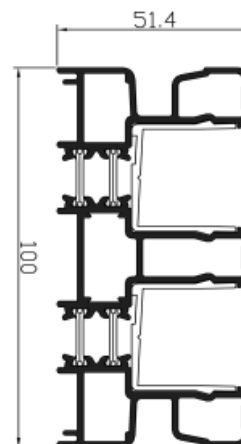
Ref. 22408 Marco tres carriles perimetral
