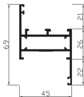
Ref. 21501 Marco ventana con tapajuntas
