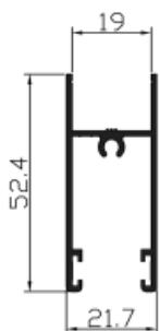
Ref. 24589 Hoja casaca para vidrio cámara
