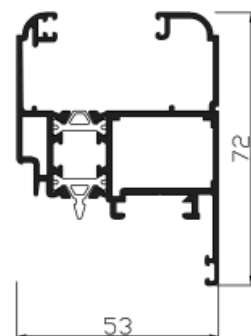
Ref. 22740 Hoja ventana vidrio directo
