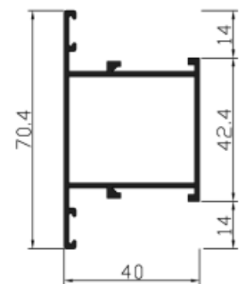
Ref 10423 Perfil travesaño
