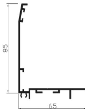
Ref. 24554 Angulo para registro 85 mm
