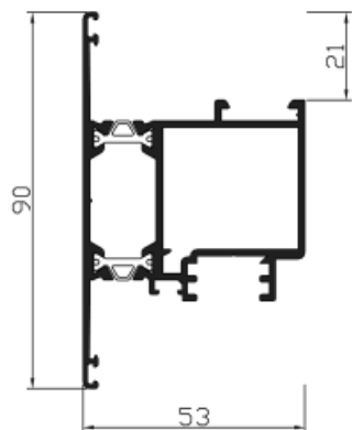
Ref. 22737 Hoja pivotante
