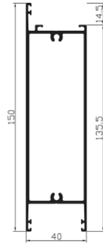
Ref. i9737 Perfil de zócalo
