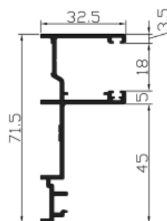
Ref. 24042 Guía de persiana 24042 *Sobre pedido
