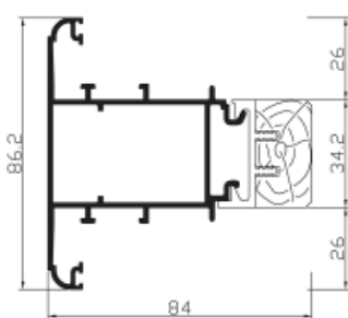
Ref 21942+7L3 Travesaño hoja
