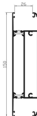
Ref. 22763 Franja vidrio directo
