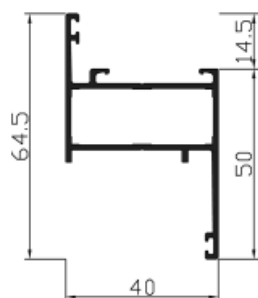
Ref. 26200 Marco con tapajuntas
