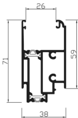
Ref. 22765 Suplemento zócalo vidrio directo
