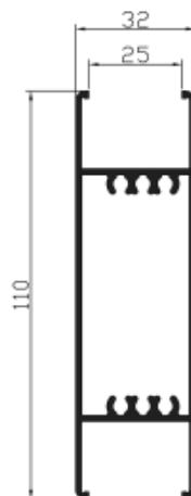
Ref. 24427 Travesaño vidrio directo
