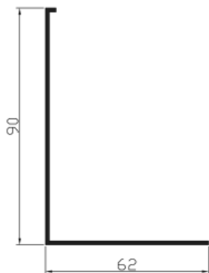
Ref. 9062 Angulo de 90x62
