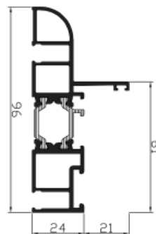
Ref. 22182 Semi rigidizador
