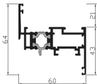
Ref 22010 Hoja ventana
