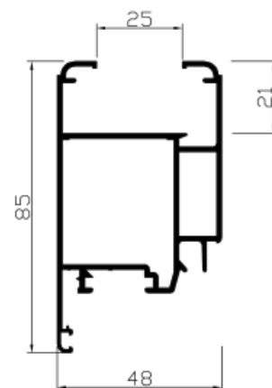
Ref. 27040 Hoja balconera vidrio directo
