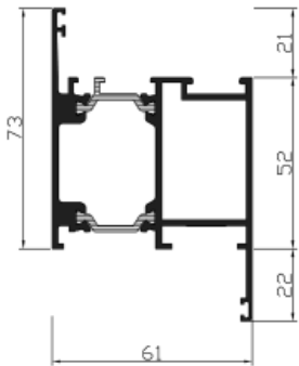
Ref. 22151 Marco puerta con tapajuntas
