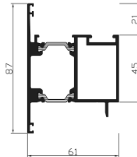
Ref. 22161 Hoja puerta apertura exterior
