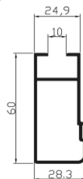
Ref. 24592 Hoja cruce para vidrio normal
