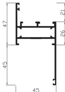
Ref. 21611 Marco con tapajunas
