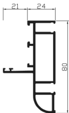
Ref. 21546 Semi rigidizador
