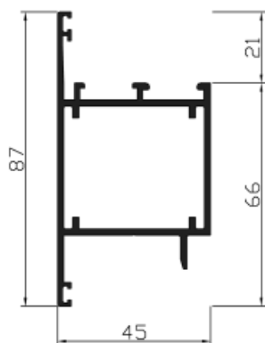
Ref. 21588 Hoja puerta apertura exterior
