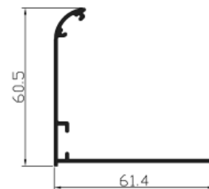
Ref. 65021 Angulo curvo
