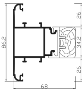
Ref 21941+7L3 Travesaño marco
