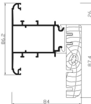
Ref 21942+7L4 Suplemento zócalo
