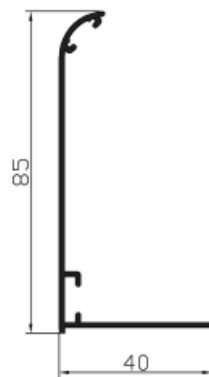
Ref. 65031 Angulo curvo.
