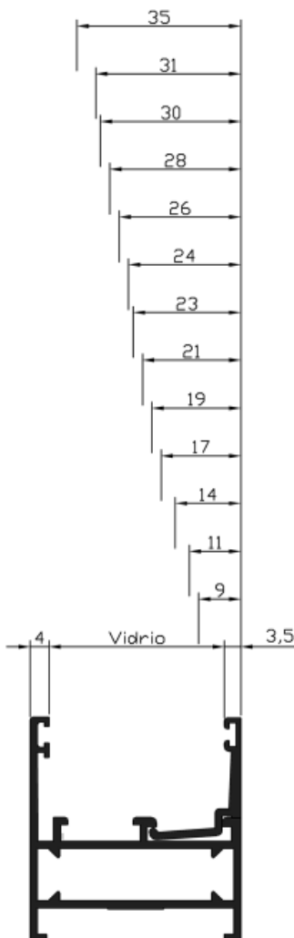
Ejemplo de tabla de aplicación de junquillos para acristalamiento. Esquema representado serie GREEN.
