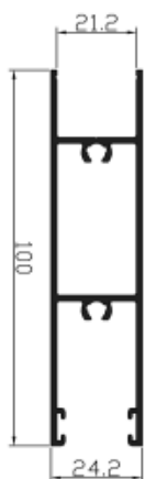
Ref. 72022 Hoja zócalo para vidrio cámara
