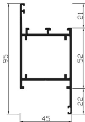
Ref. 21508 Marco puerta con tapajuntas
