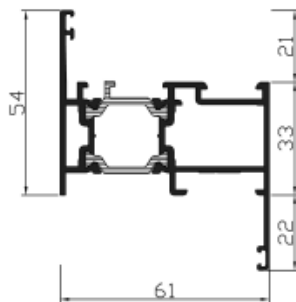
Ref. 22156 Marco ventana con tapajuntas
