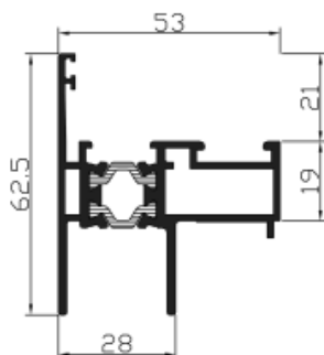
Ref 22310 Marco ventana
