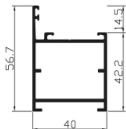
Ref. 30066 Marco puerta sin tapajuntas
