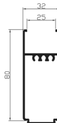
Ref. 24428 Suplemento zócalo vidrio directo
