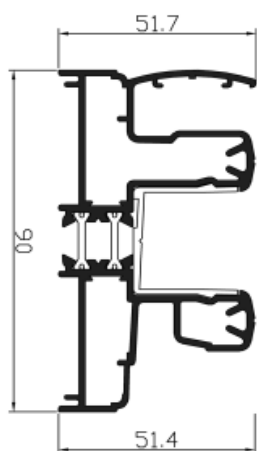
Ref. 22401 Marco 90 mm corte perimetral o corte recto
