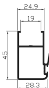
Ref. 24590 Hoja cruce para vidrio cámara
