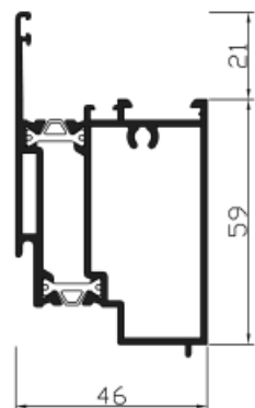
Ref. 22764 Suplemento zócalo
