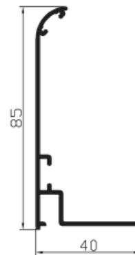
Ref. 65032 Angulo para registro.
