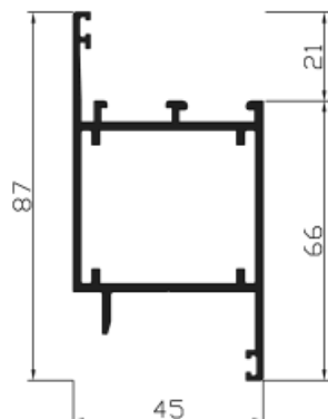
Ref. 21589 Hoja puerta apertura interior
