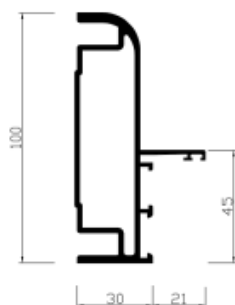
Ref. 24524 Semi rigidizador
