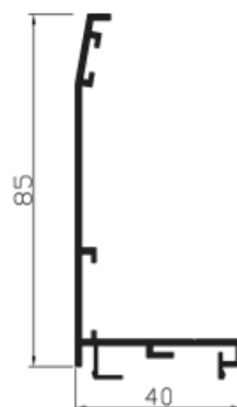
Ref. 27600 Angulo de registro de 85 mm
