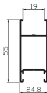
Ref. 24591 Hoja lateral para vidrio cámara
