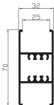
Ref. 24426 Travesaño vidrio directo
