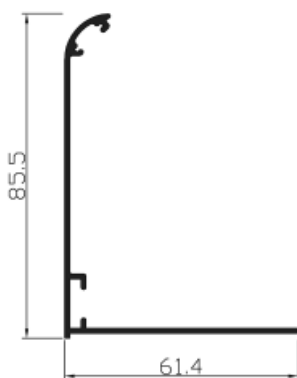
Ref. 65019 Angulo curvo.
