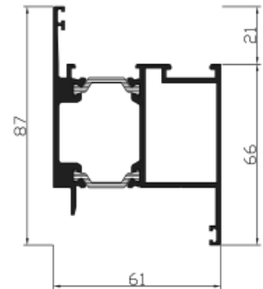
Ref. 22162 Hoja puerta apertura interior
