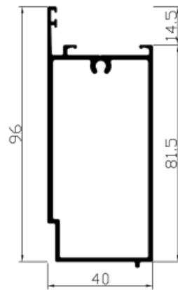
Ref. 26194 Suplemento zócalo para hoja perimetral
