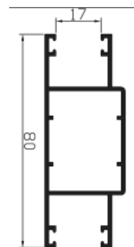
Ref. 7311 Guía de persiana doble 7311
