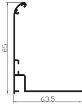
Ref. 65022 Angulo para registro.
