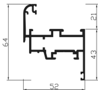
Ref. 21513-24540 Hoja ventana con punto redondo * Consultar stock
