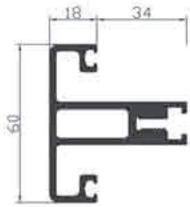
Ref. 21107 Travesaño
