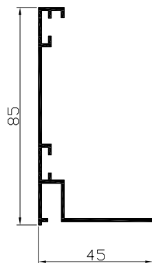
Ref. 65042 Angulo para registro.
