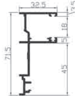
Ref. 2402 Guia de persiana 2402 *Sobre pedido
