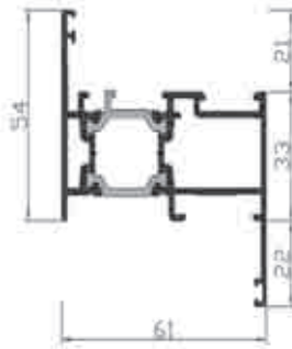
Ref 22052 Marco ventana con tapajuntas *Consultar stock
