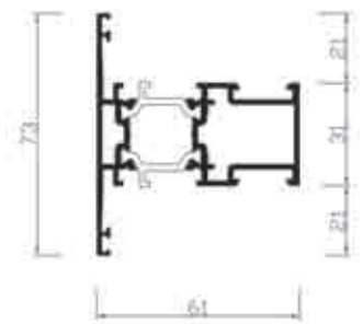
Ref 22093 Travesaño
