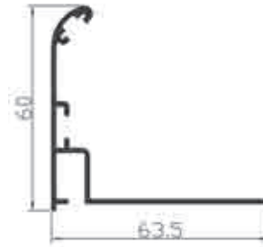
Ref. 65023 Angulo para registro
