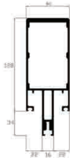
Ref. 21109 Rigidizador 162 mm.
