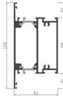
Ref 22070 Travesaño / franja
