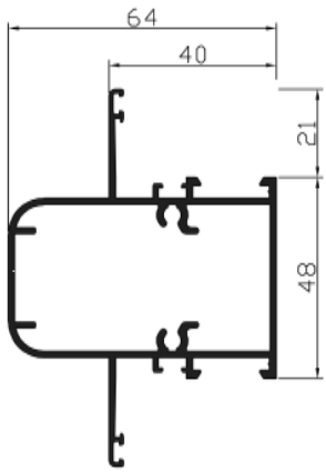
Ref. 27067 Rigidizador
