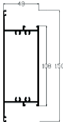
Ref. 27074 Zócalo
