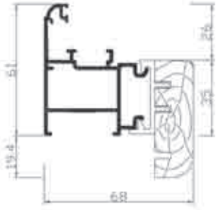
Ref. 21901+7L2 Marco ventana con tapajuntas
