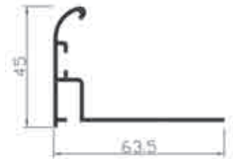
Ref. 65024 Angulo para registro.
