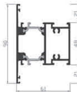
Ref 22091 Travesaño
