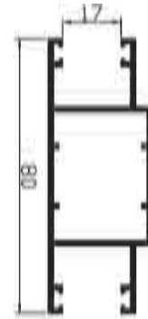
Ref. 7311 Guia de persiana doble 7311
