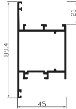
Ref. 21645 Hoja balconera apertura exterior
