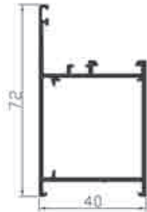
Ref. 27002 Marco puerta sin tapajuntas
