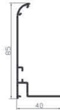
Ref. 65032 Angulo para registro.
