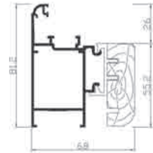
Ref. 21902+7L2 Marco puerta
