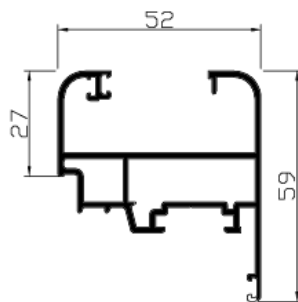
Ref. 24539 Hoja vidrio directo * Consultar stock
