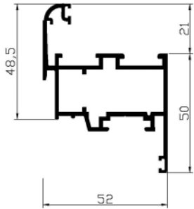
Ref. 21640 Hoja punto redondo resalte
