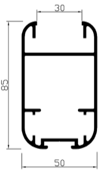
Ref. 121685 Hoja reforzada
