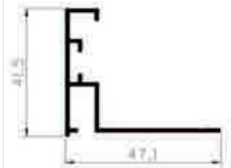
Ref. 65041 Angulo para registro.
