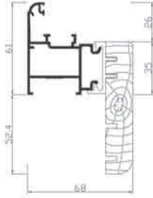
Ref. 21901+7L4 Marco ventana con tapajuntas
