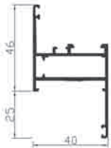
Ref. 27001 Marco ventana con tapajuntas.
