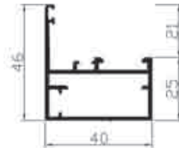
Ref. 27003 Marco ventana plano.
