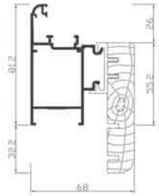
Ref. 21902+7L4 Marco puerta con tapajuntas
