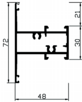
Ref. 27073 Travesaño
