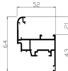
Ref. 24540 Hoja ventana de punto redondo
