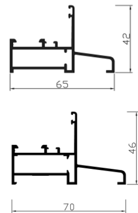
Ref. 65030 - 70009 Perfil para fijos compatibles con corredera P70
