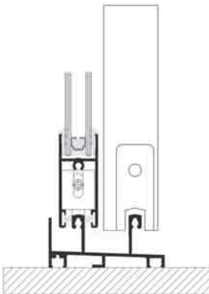
Corredera Samblex 65i
