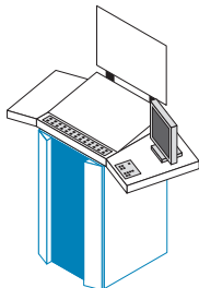
Puestos de mando por ej. para impresoras, compuestos por: ● Caja IW ● Superficie de trabajo individual, así como componentes.
