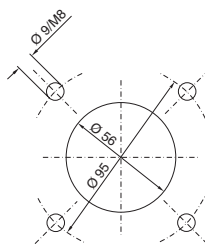
Escotadura de montaje
