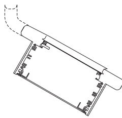
Profundidad de montaje 105 mm para teclados empotrables
