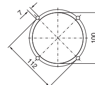
Escotadura de montaje Caja CP-XL
