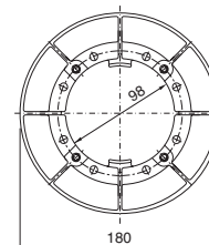
Escotadura de montaje Caja CP-XL
