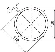
Sección de montaje de la caja CP-XL
