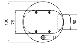
Escotadura de montaje Caja CP-L Ø 130 mm
