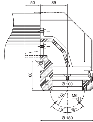
Escotadura de montaje Caja CP-XL
