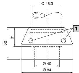
1 Tornillo de apriete
