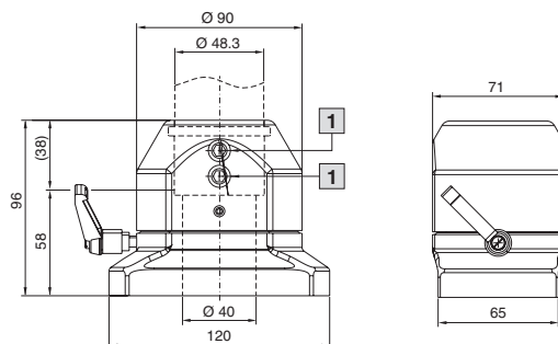
1 Tornillo de seguridad
