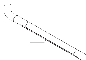
Prof. 27 mm con conducto para cables, flexible, para teclados de sobremesa
