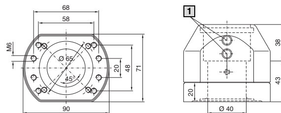
1 Tornillo de apriete
