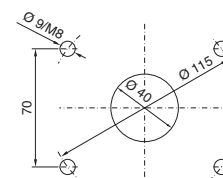
Escotadura de montaje
