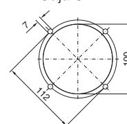
Escotadura de montaje Caja CP-XL
