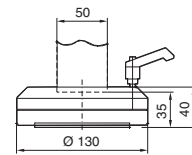
Escotadura de montaje Caja CP-L, Ø 130 mm
