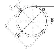
Escotadura de montaje Caja CP-XL
