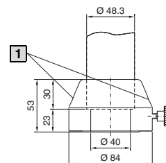
1 Tornillo de apriete
