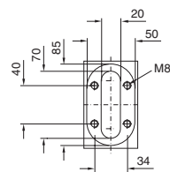
Vista A
