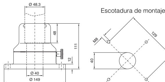
2 Fijación exterior CP 6663.400
