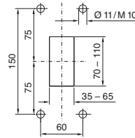
Escotadura de montaje
