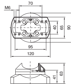
Escotadura de montaje Caja CP-L, □ 120 x 65 mm
