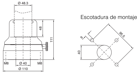
2 Fijación exterior CP 6663.400
