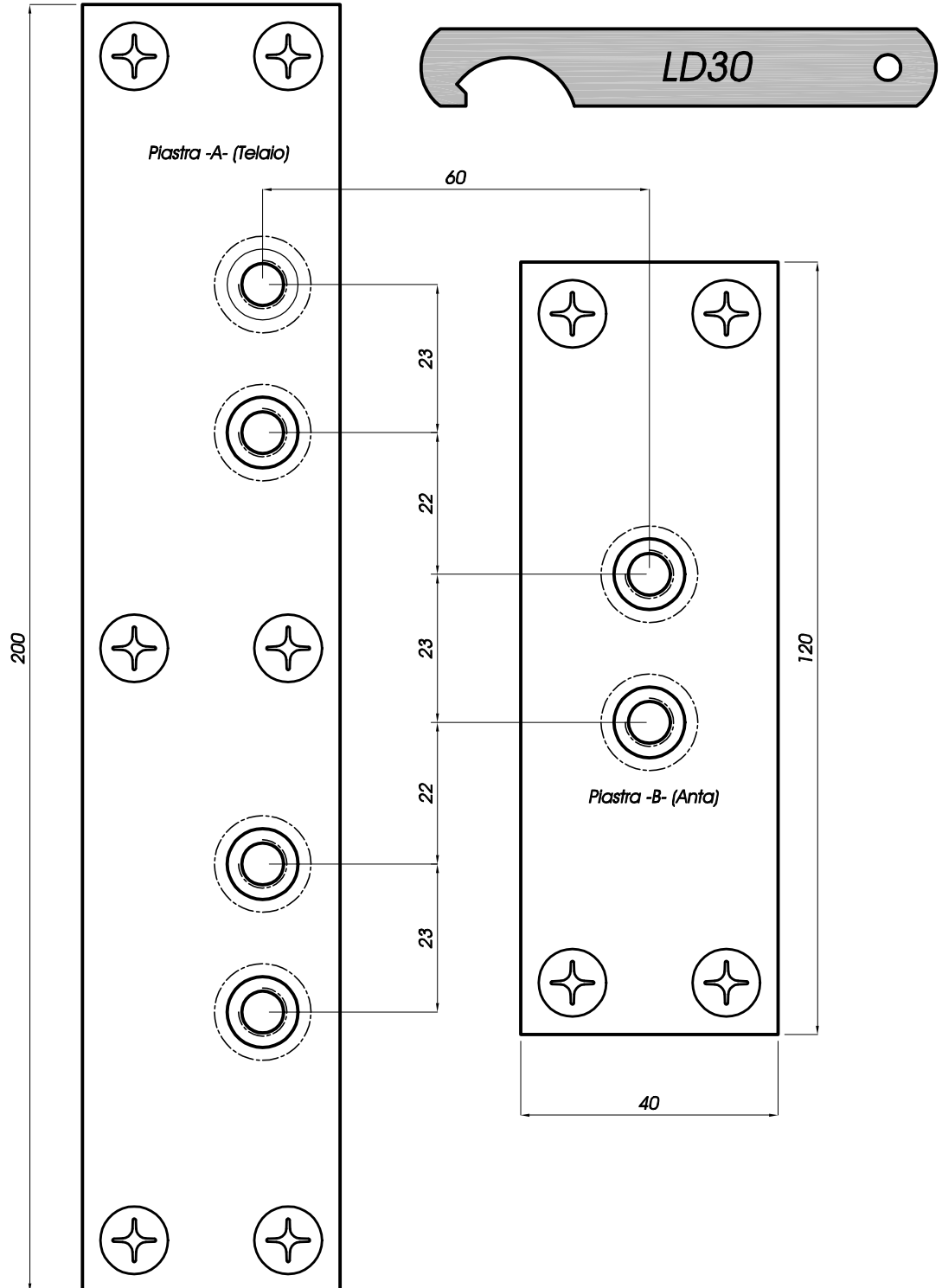
Nuova cerniera regolabile nelle tre direzioni con chiave LD30
