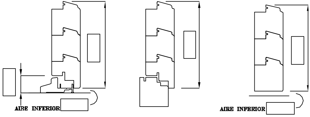
ZOCALO DE PUERTAVENTANA ZOCALO DE PUERTAVENTANA ZOCALO CON PARAFRIO EVENTUAL DIFERENTE
