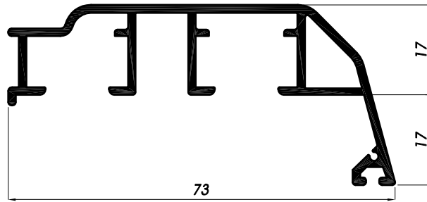
LA261 - Anta legno 113mm
