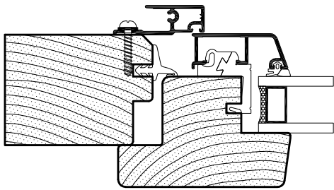
LIGHT/45 senza guida
