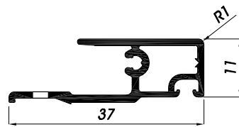
LA271 Montanti + superiore
