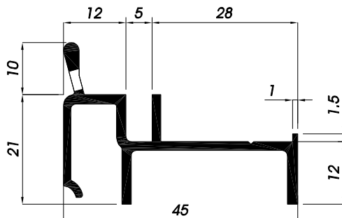
PA216 soglia 31mm
