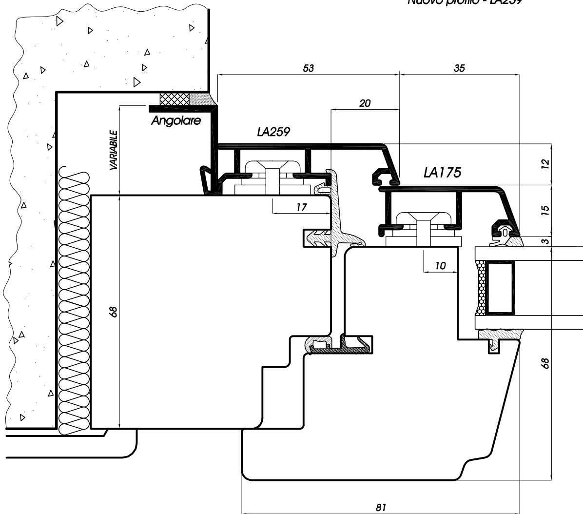
Nuovo profilo - LA259
