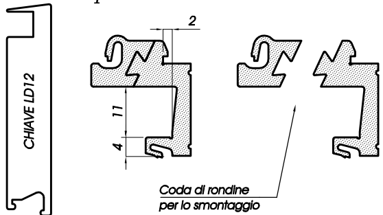
LC24 – Clips a scatto senza vite per battuta vetro 20mm
