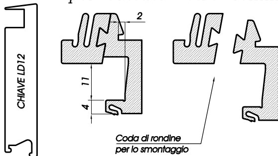
LC31 – Clips a scatto senza vite per battuta vetro 20mm
