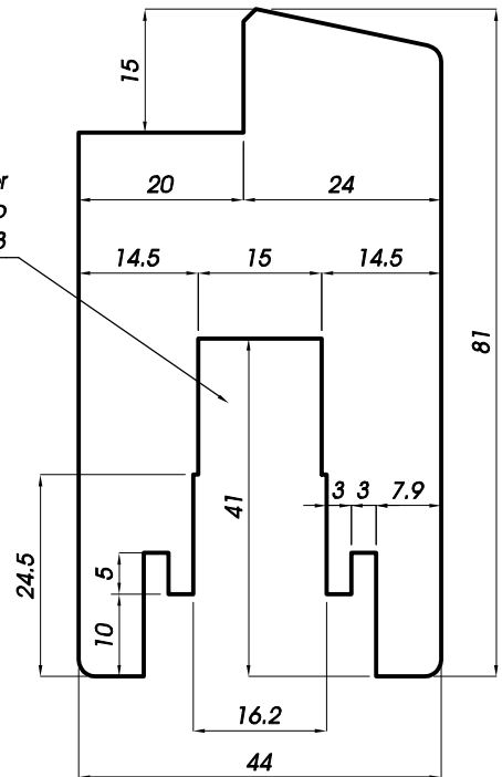
Sezione anta traverso inferiore
