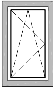
Fin. 1 ante L= 410-1200mm H= 485-1800mm
