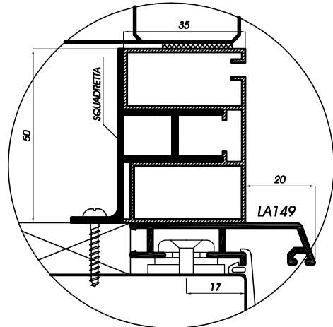
Variante senza guida avvolgibile
