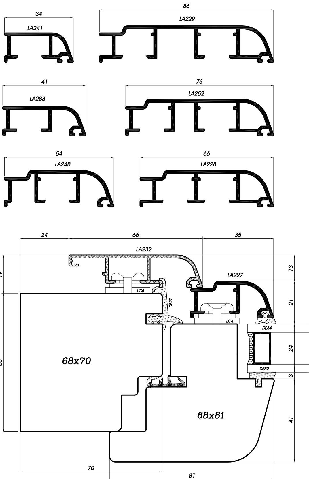
Sezioni orizzontali battenti Horizontalschnitte Flügel Secciones horizontales hojas Coupes horizontales vantaux Horizontal section of the wings
