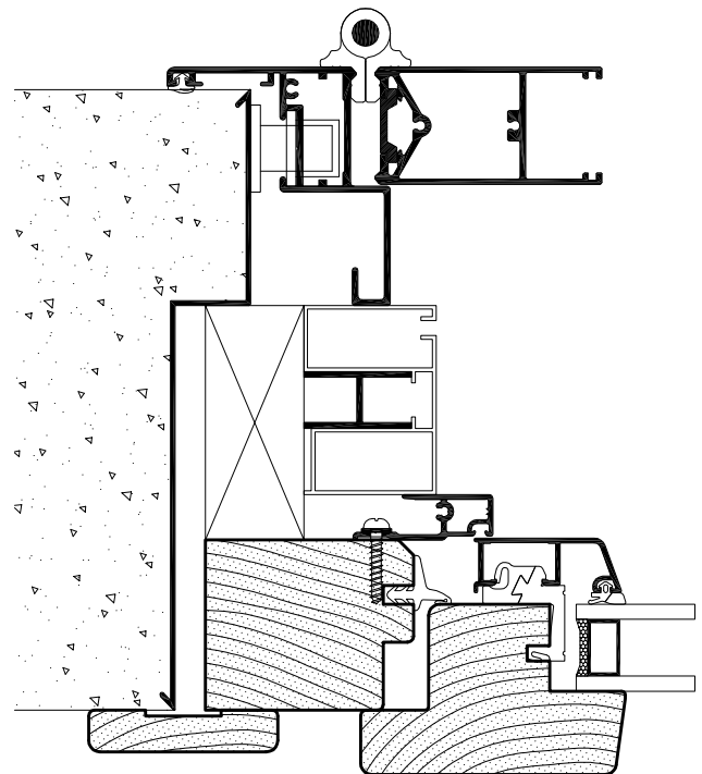
LIGHT/45 Monoblocco zanzariera + scuretto 30mm
