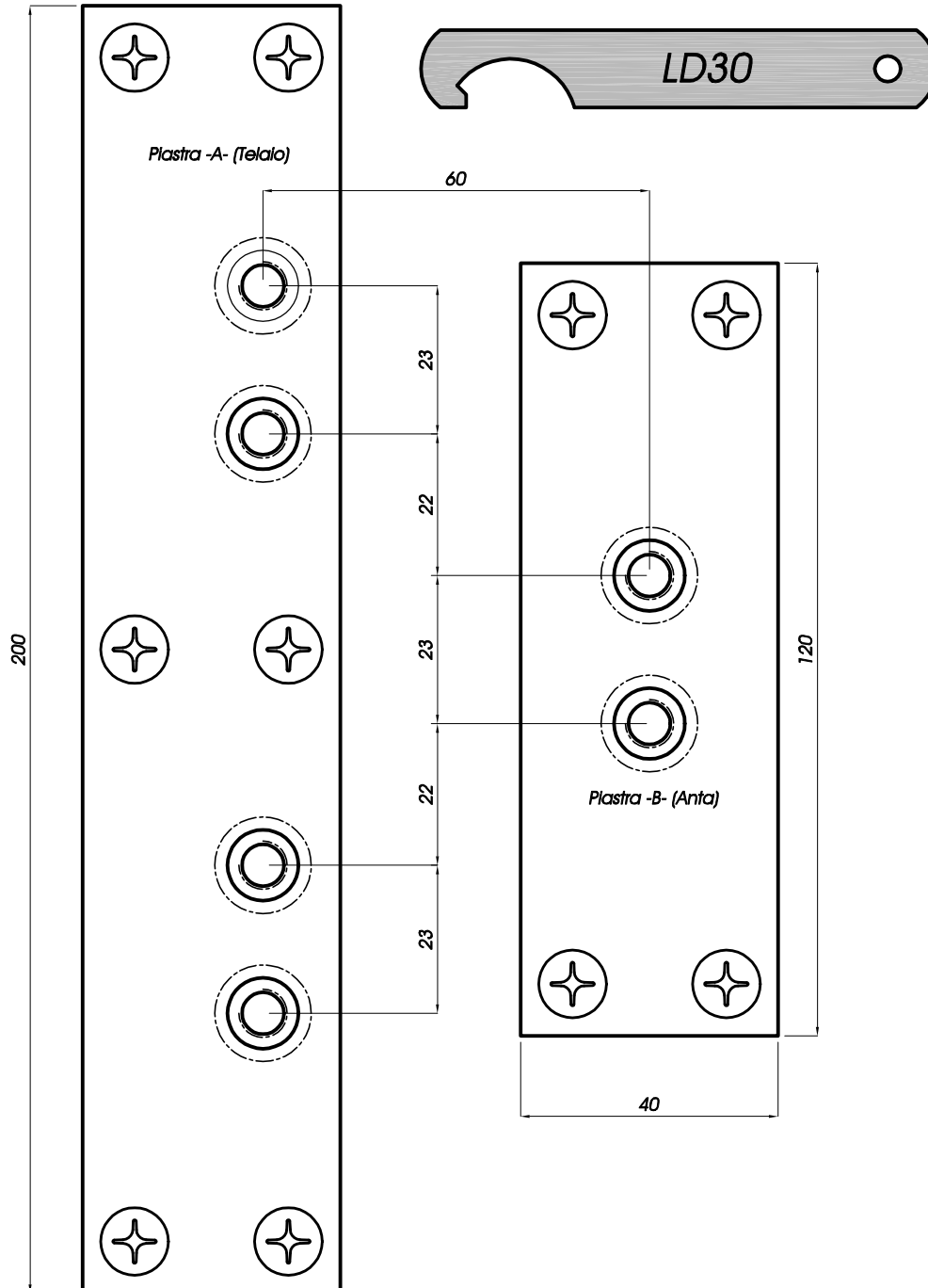
Nuova cerniera regolabile nelle tre direzioni con chiave LD30
