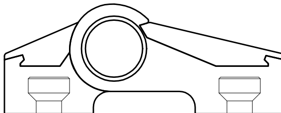
Nuova cerniera regolabile nelle tre direzioni con chiave LD30
