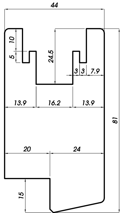
Sezione anta traverso superiore
