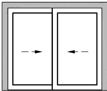
Fin. Scorrevole L= 1300-2800mm H= 800-1800mm
