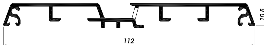
LA274C con asole per scarico acqua
