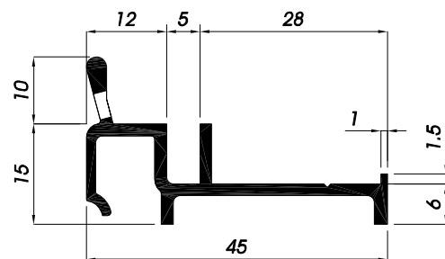
PA220 soglia 25mm
