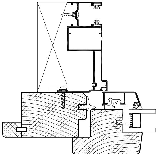
LIGHT/45 Monoblocco zanzariera + guida
