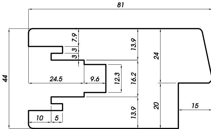
Sezione anta montante laterale
