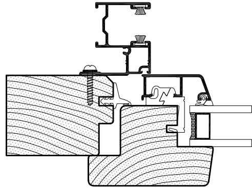
LIGHT/45 con guida
