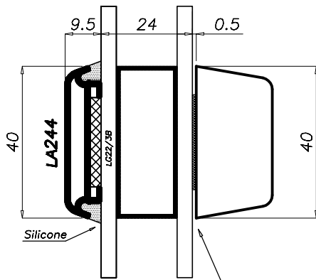
NASTRO BIADESIVO LCN19
