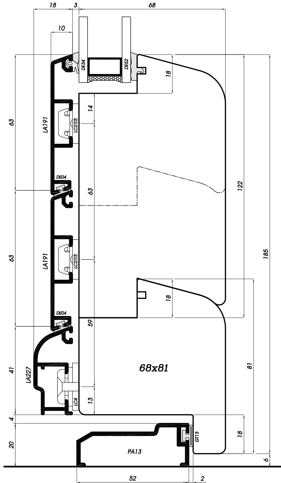
Sezione verticale traverso inferiore portafinestra con PA13 Vertikalschnitt Balkontür quer unten mit PA13 Sección vertical travesaño inferior puertaventana con PA13 Coupe verticale traverse inférieure porte-fenêtre avec PA13 Vertical section of the lower ledger for window-door with PA13
