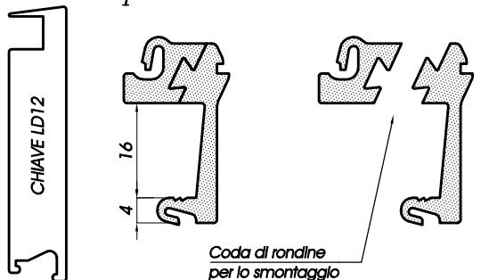
LC13 – Clips a scatto senza vite per battuta vetro 20mm
