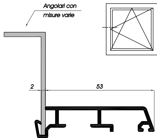
Nuovo profilo - LA259
