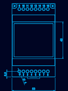
16 conexiones / connections
