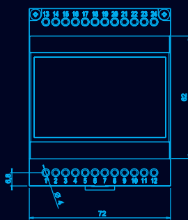
24 conexiones / connections
