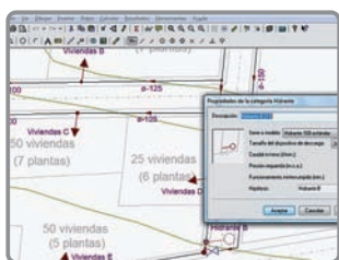
Redes de abastecimiento de agua
