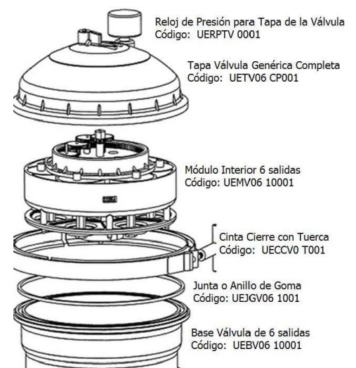
Inside Module for Water Valve 6 ports Módulo Interior Válvula Distribuidora 6 salidas Module Vanne de Commande 6 sorties
