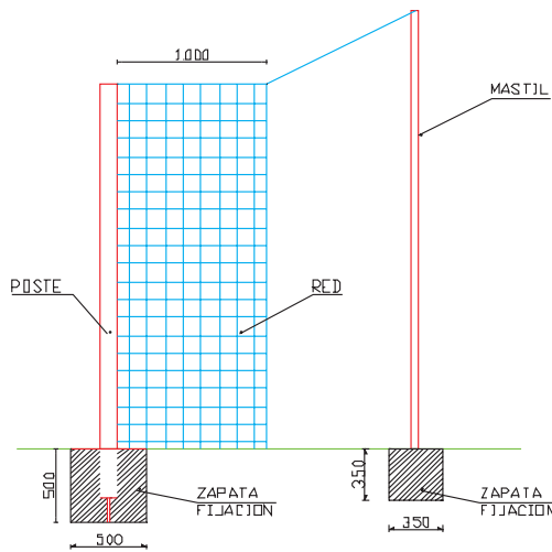
PORTERIA FIJA PF 702
