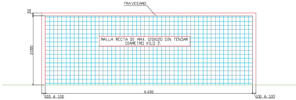
PORTERIA TRASLADABLE PF 721
