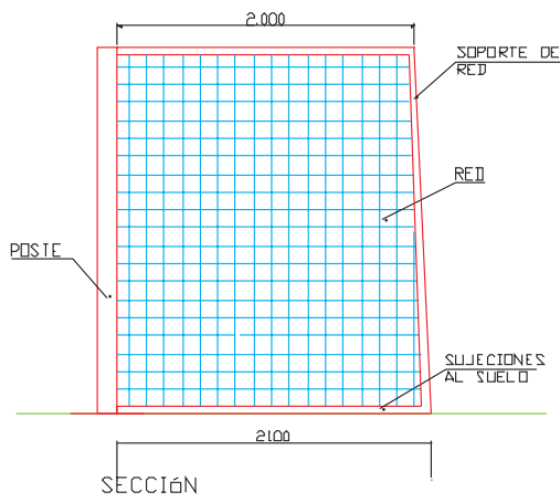
PORTERIA FIJA PF 702
