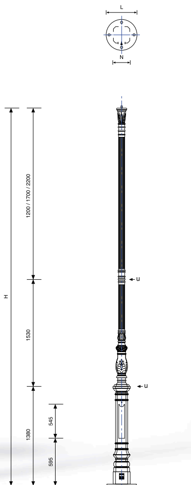
Cast Iron Fundición de hierro
