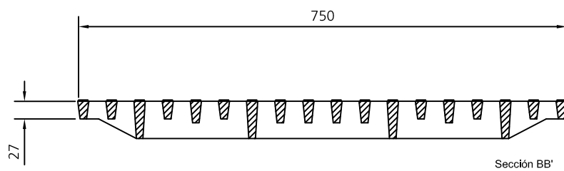
Sección BB'
