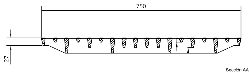
Sección AA'
