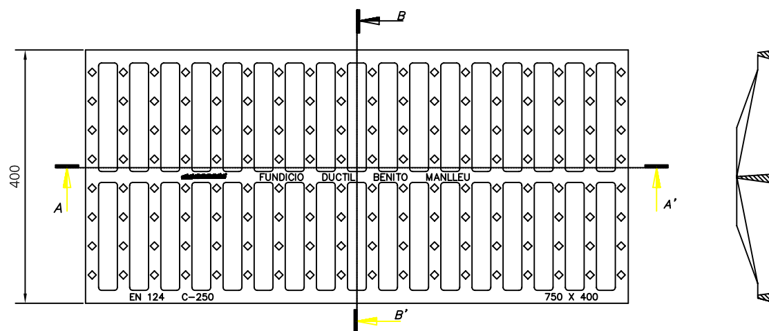
Sección BB'
