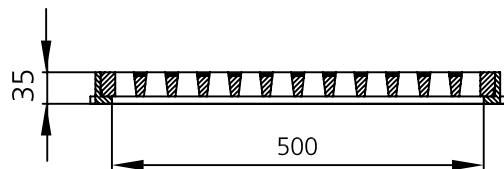
Sección AA'
