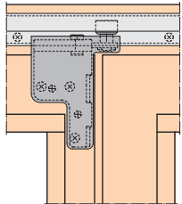
Corte con carros en parte inferior 1:2,5
