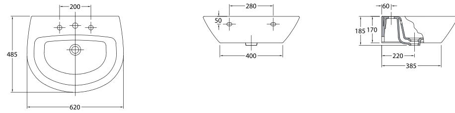
28020 Lavabo Jazz de 62 x 48,5 cm. Con rebosadero y juego de fijación. Válido para mural, pedestal, semipedestal o sobre-encimera.
