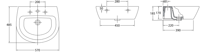
28030 Lavabo Jazz de 57 x 48,5 cm. Con rebosadero y juego de fijación. Válido para mural, pedestal, semipedestal o sobre-encimera.
