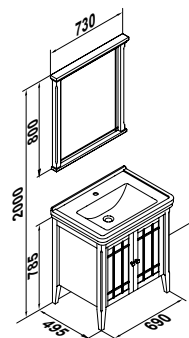
MUEBLE BASE PARA LAVABO 75 cm. # 38650 ESPEJO de 73 x 80 PARA MUEBLE BASE LAVABO # 38670 VANITY UNIT FOR WASHBASIN - 73 x 80 MIRROR FOR VANITY UNIT
