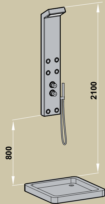
Cotas conexión de fontanería / Plumbing connections
