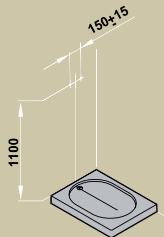
Cotas conexión de fontanería / Plumbing connections
