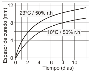
Diagrama 1: Velocidad de curado del Sikaflex®-222 UV
